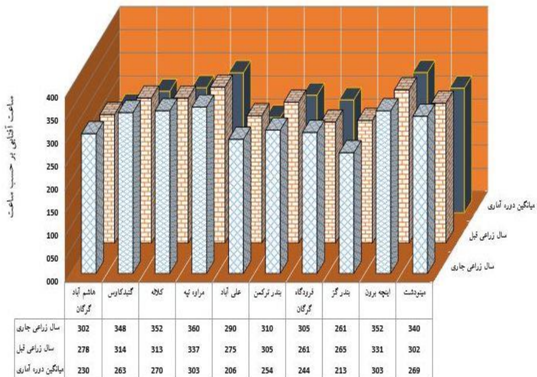
شکل ۴: مقایسه نوسانات مجموع ساعت آفتابی تیر (ساعت)
