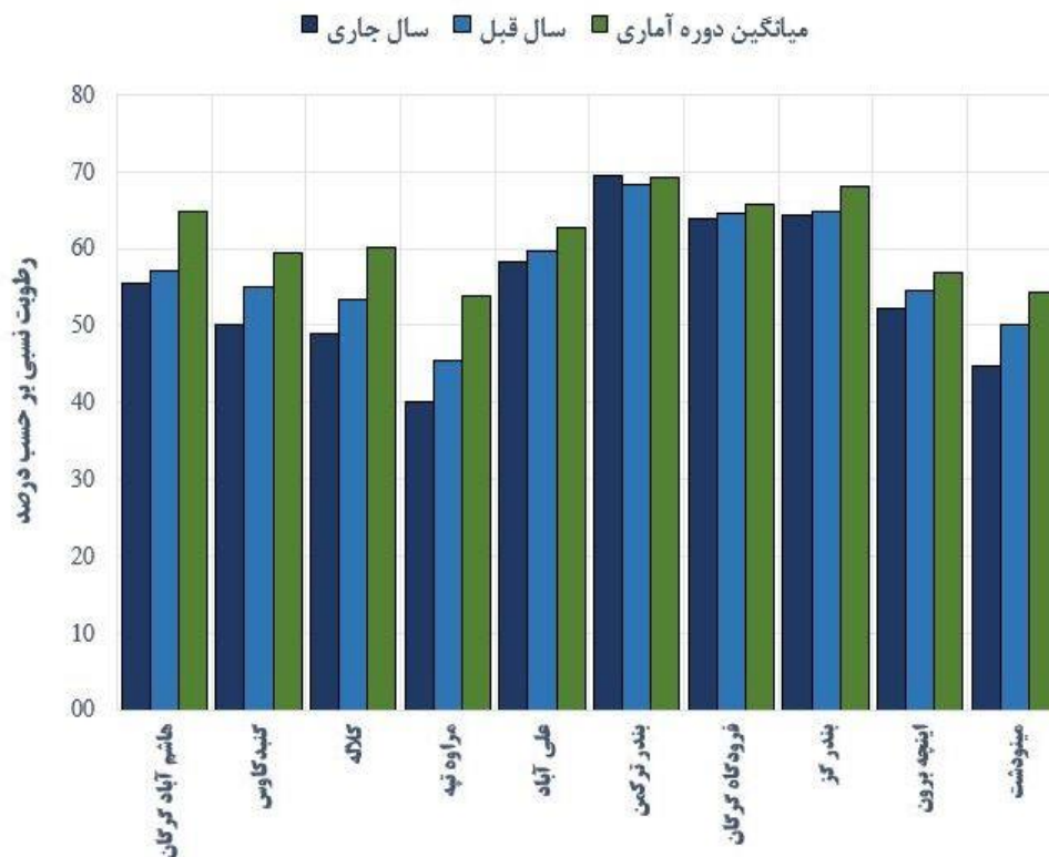
شکل ۳: مقایسه نوسانات میانگین رطوبت نسبی هوا خرداد ماه
