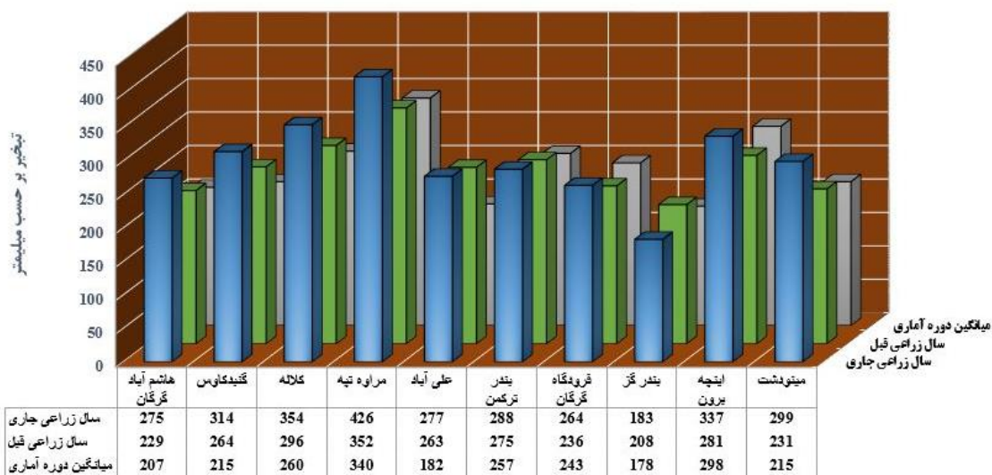
شکل ۵: مقایسه نوسانات مجموع میزان تبخیر خرداد (میلی متر)
