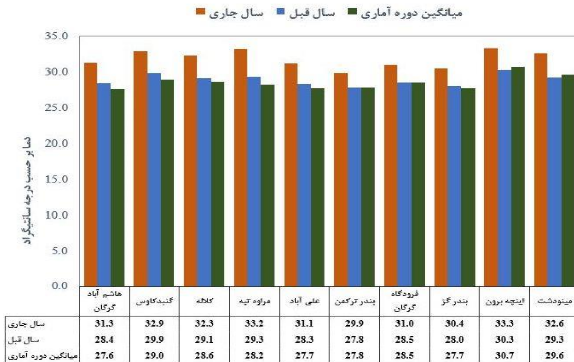
شکل ۲: مقایسه میانگین دمای هوا خرداد
