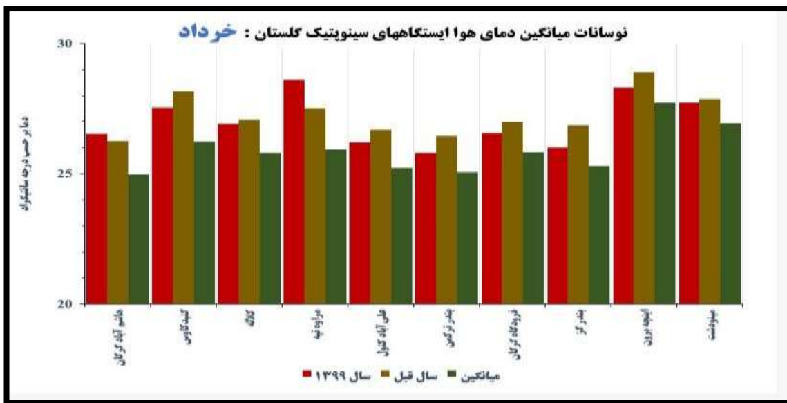
شکل ۲: مقایسه میانگین دمای هوا خرداد ماه
