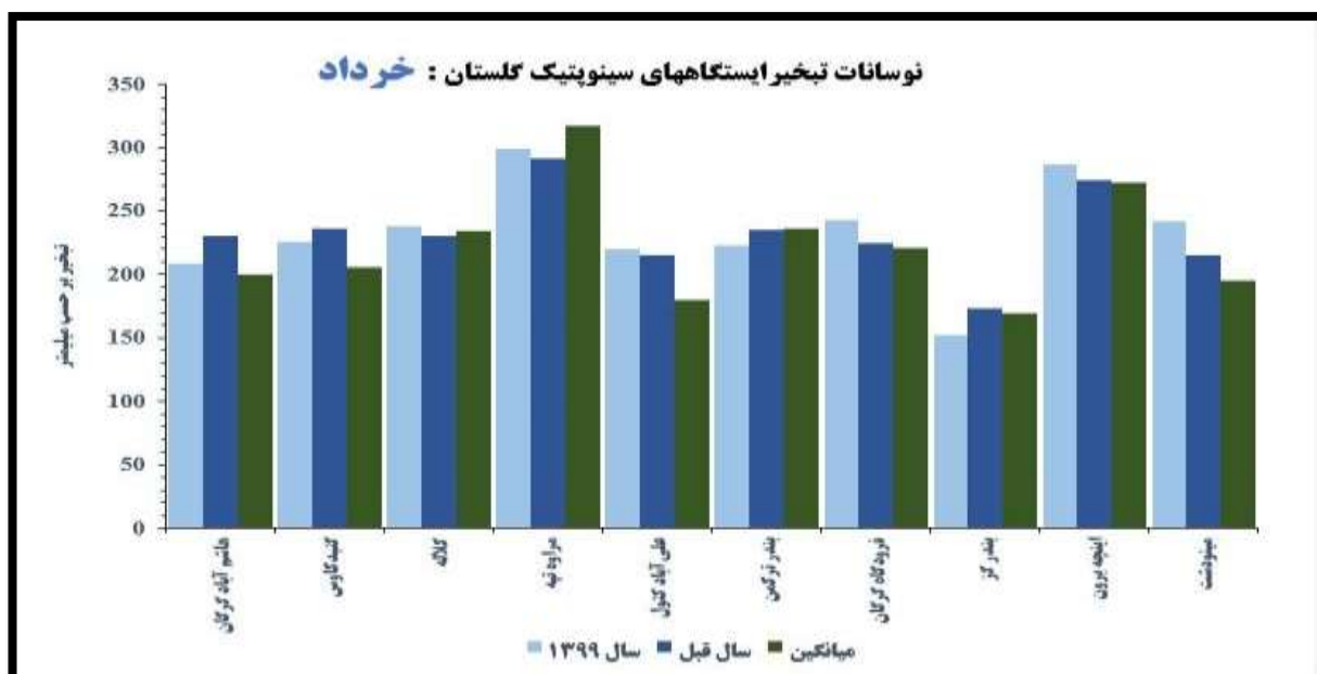
شکل ۵ : مقایسه نوسانات مجموع میزان تبخیر خرداد ماه (میلی متر)
