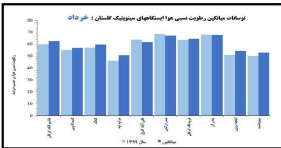
شکل ۳: مقایسه نوسانات میانگین رطوبت نسبی هوا خرداد ماه
